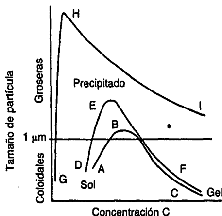
Fig. 20-1. Efecto de la concentración del material precipitante y del envejecimiento en el tamaño de las partículas. 5,13 Las curvas ABC, DEF y GHI corresponden al envejecimiento creciente. Ambos ejes están en escala logarítmica.
