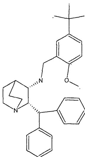
Ilustración 1. Maropitant
