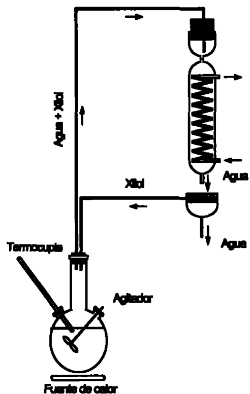
Figura 1. Montaje experimental.
