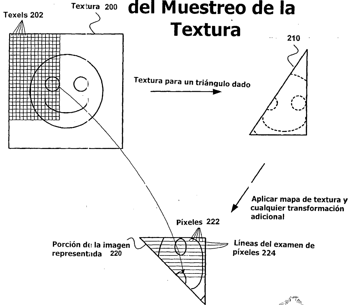
FIG. 1 - Técnica Anterior
