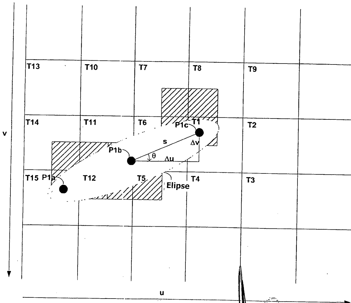
FIG. 2D - Técnica Anterior Filtrado Anisotrópico
