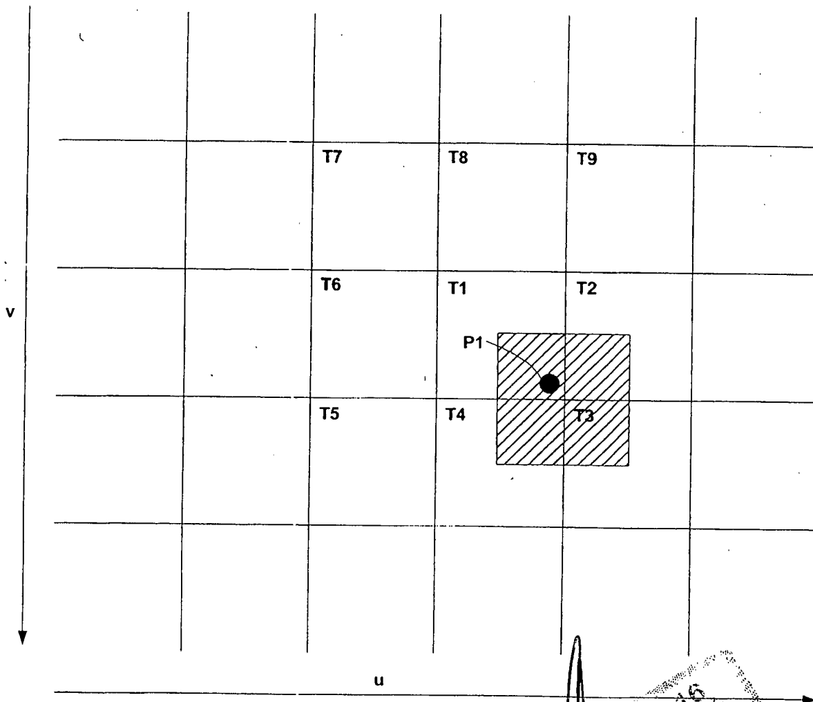
FIG. 2B - Técnica Anterior Filtrado Bilinear
