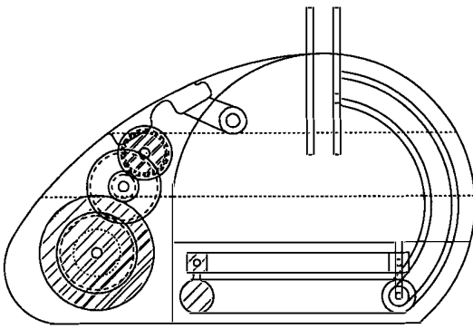
Corte lateral izquierdo
