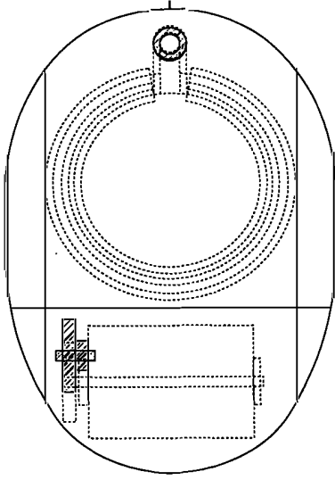
Corte inferior
