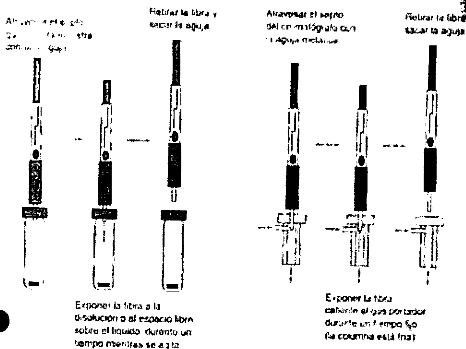
Figura 24.20 Toma de muestra mediante microextracción en fase sólida y desorción de analito de la fibra recubierta, para su introducción en un cromatógrafo de gases. (Tomado de Supercritical Chromatography , Product Catalog, Belleronte PA.)
