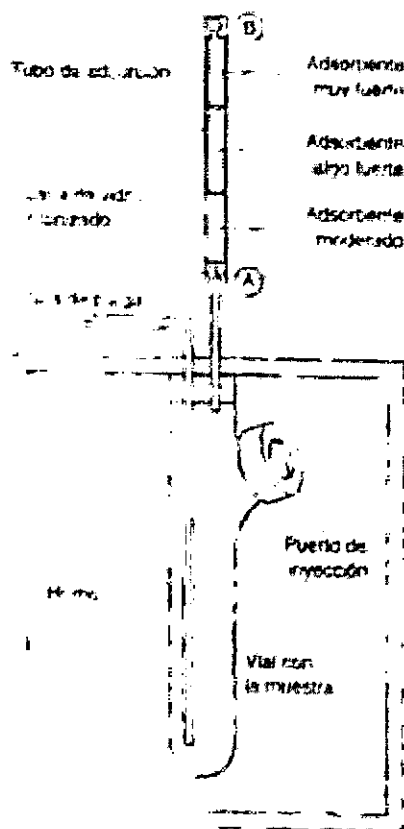
Figura 24.22 Aparato de purga y trampa para extraer sustancias volátiles de un líquido o sólido mediante una corriente de gas.
