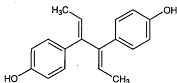
( trans-trans )-form
