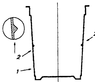
FIGURA 1 ENVASE CON APLICACIÓN DEL MODELO DE UTILIDAD. EJEMPLO CON UN REFUERZO ANULAR
