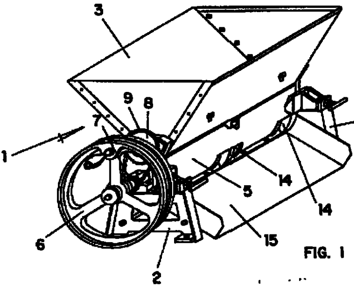
Figura 1 del documento ES 1 007 513 (D1)
