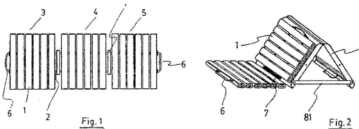
Fig. 1 y 3 del documento EP 0 357 851 (D1)
