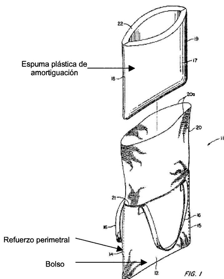
Fig. 1 del documento US 4.185.673 (D1)
