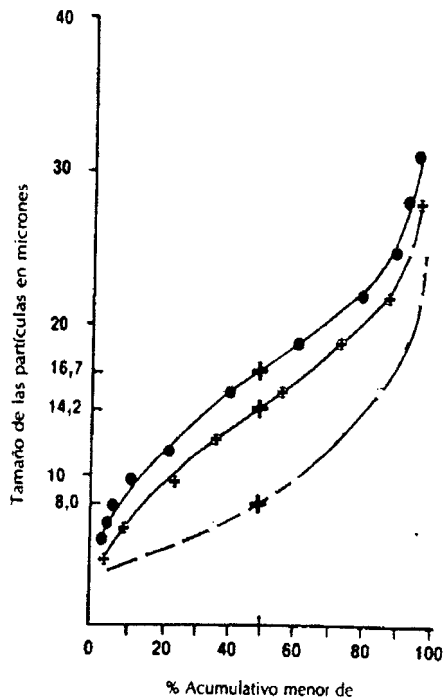
Fig. 76-2. Distribución del tamaño de partículas de cuentas de vidrio NBS expresada en términos de O = cantidad de partículas; ● = peso de las partículas; ⊗ = superficie de las partículas.
