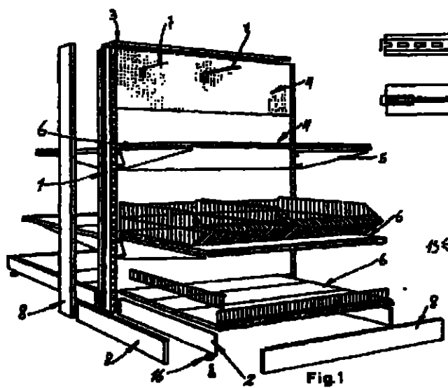
Figura 1 del documento ES 0227 351 (D1)
