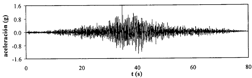
Registro de aceleración R3
