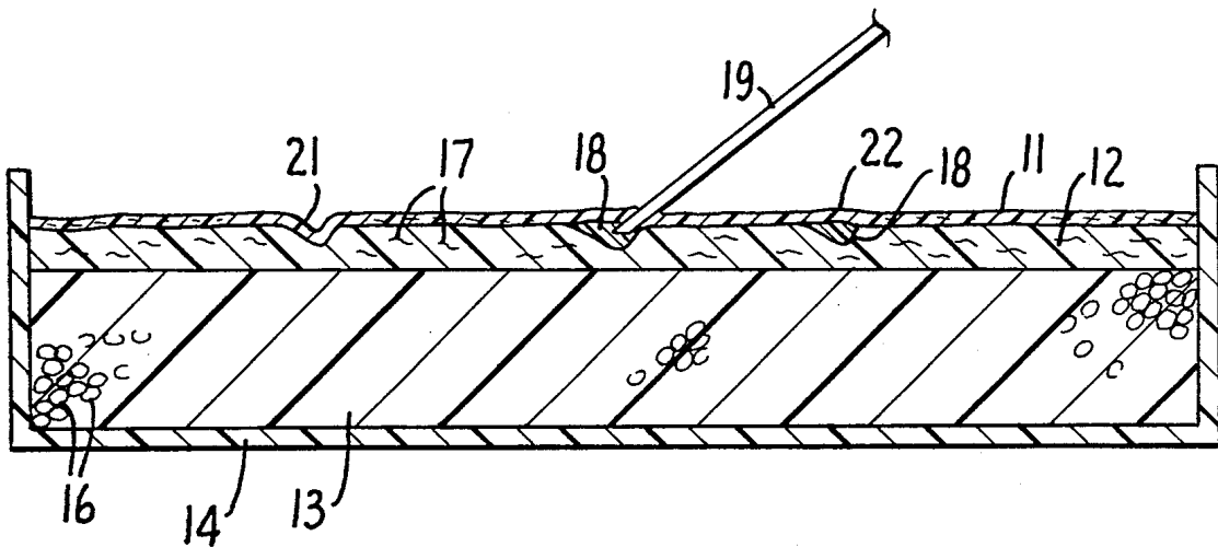
Fig. 2 del documento US 4,481,001
