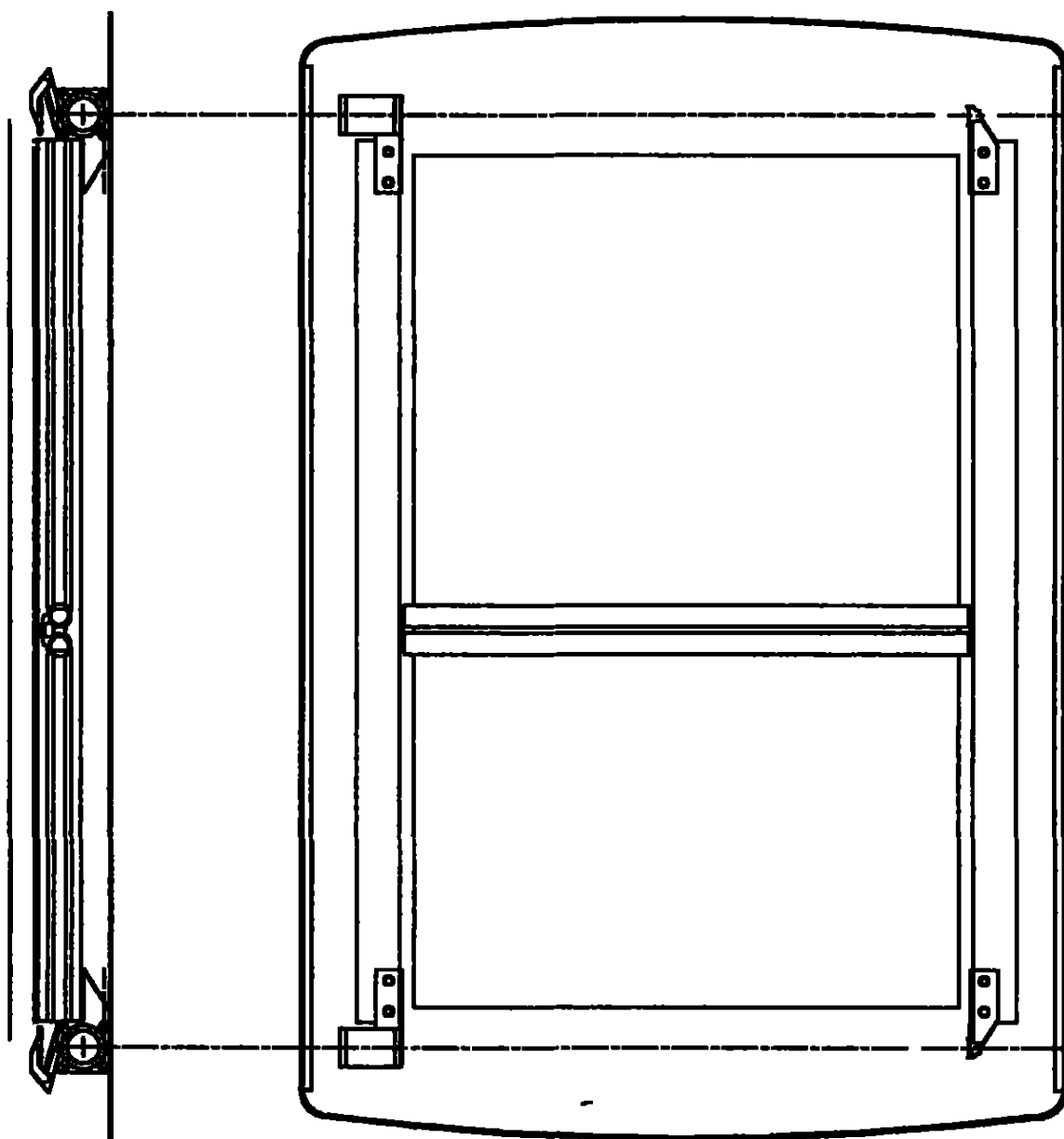
CORTE LONGITUDINAL
