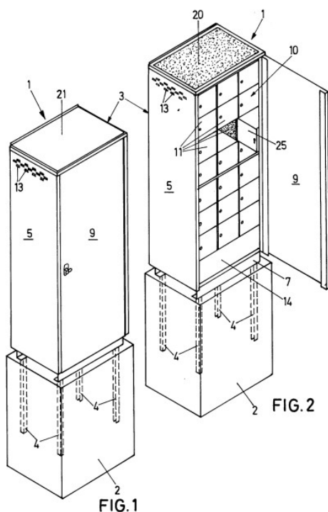
Figura 3 de D2 US 5758937
