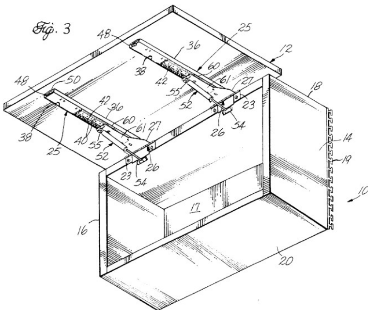
Figura 3 de D2 US 5758937
