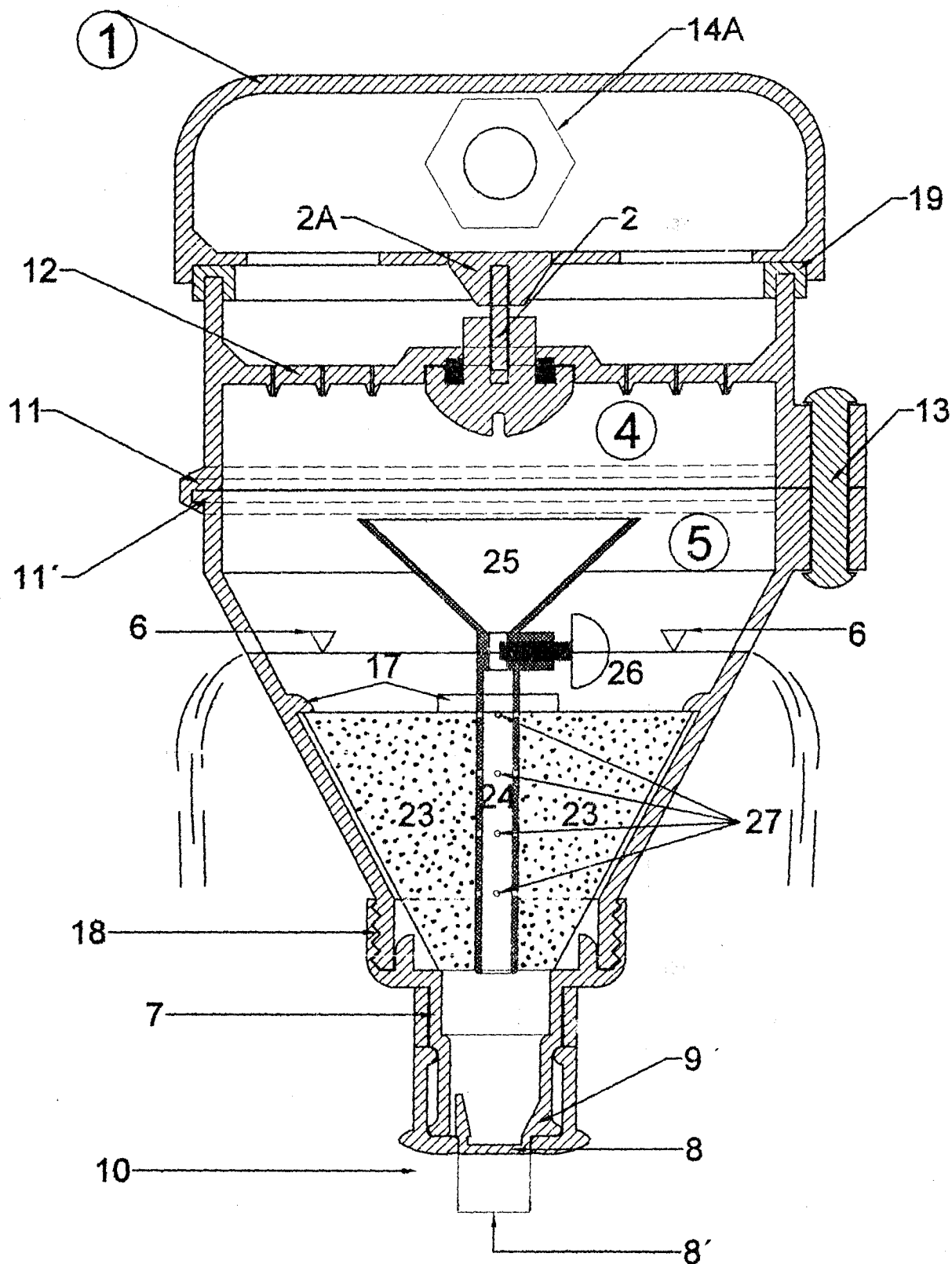
FIGURA 8 CORTE A-A' DOSIFICADOR PARA ESCENCIA EMULSIONADA DUCHA TERAPÉUTICA ESCALA 1:1
