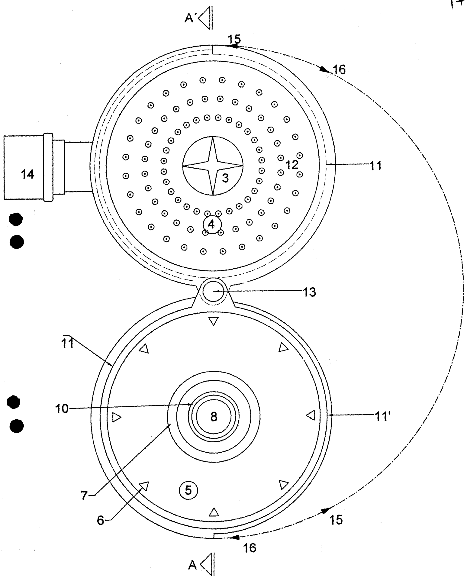
FIGURA 4A VISTA INFERIOR CONVERTIDOR TERAPÉUTICO DESPLEGADO ESCALA 1:1
