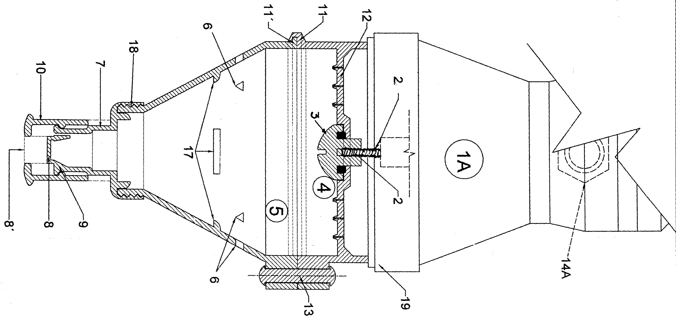
FIGURA 3A CORTE A-A' CONVERTIDOR TERAPÉUTICO (como accesorio de ducha electrica instantanea)
