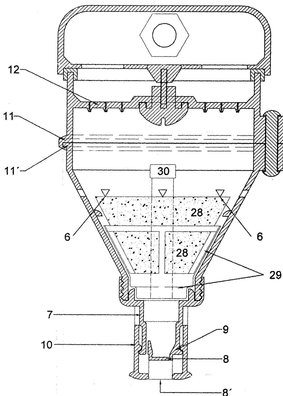
FIGURA 9 PRESENTACION OPCIONAL DE ESCENCIAS SOLIDAS PARA HIDROTERAPIA ESCALA 1:1
