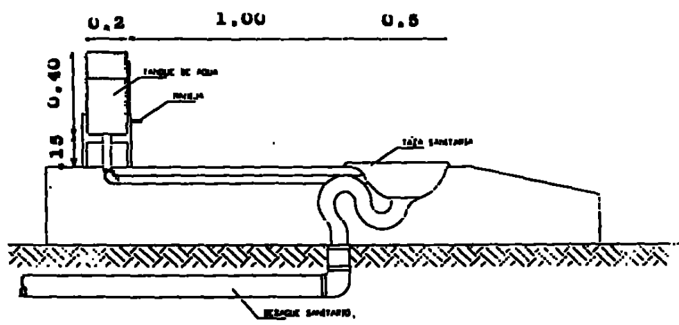
CORTE A-A
