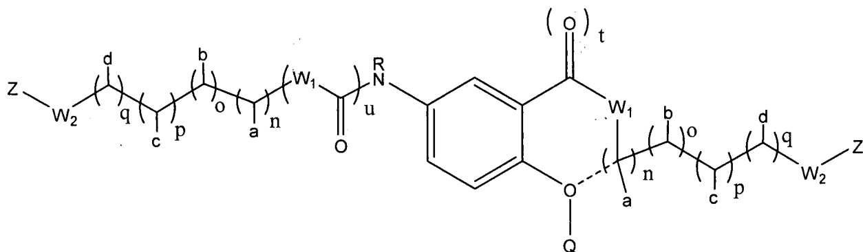
Fórmula III
