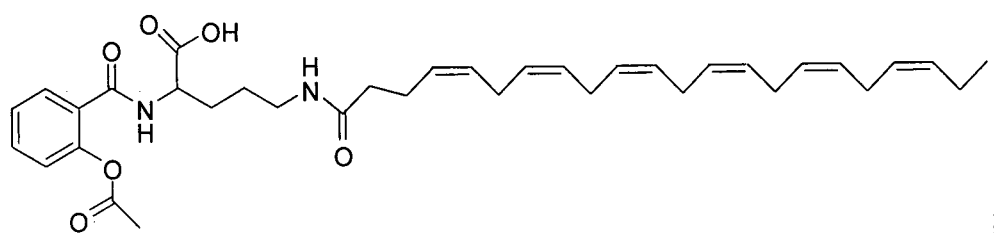
Ic-7
