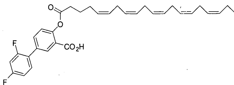
IVa-2
