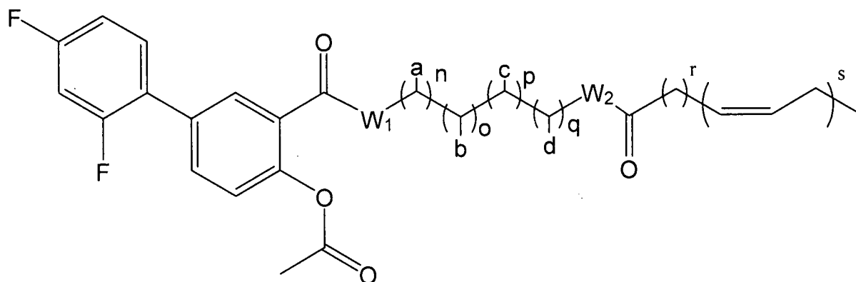
Fórmula IVb
