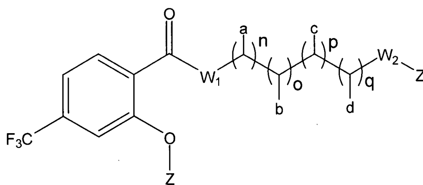
Fórmula VIc'
