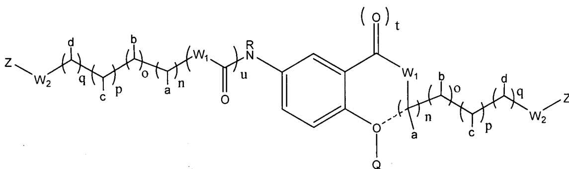
Fórmula III
