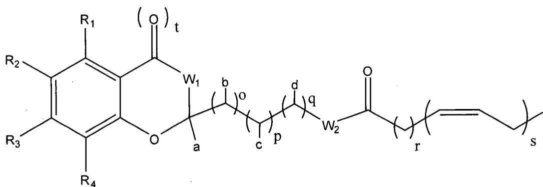
Fórmula If
