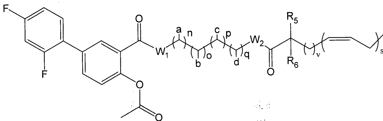
Fórmula IVb'
