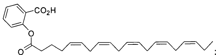
Ia-2
