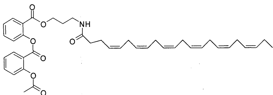
Ib-1
