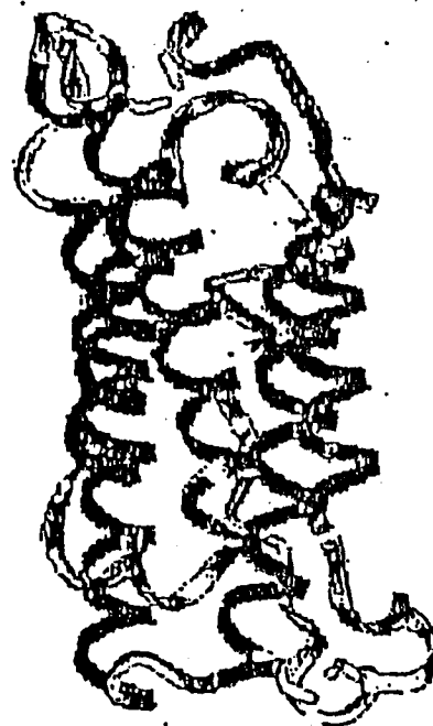
IFNα
