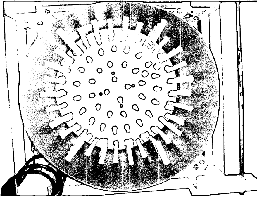
PLATO GIRATORIO CON DEDOS DE CAUCHO SUAVES
