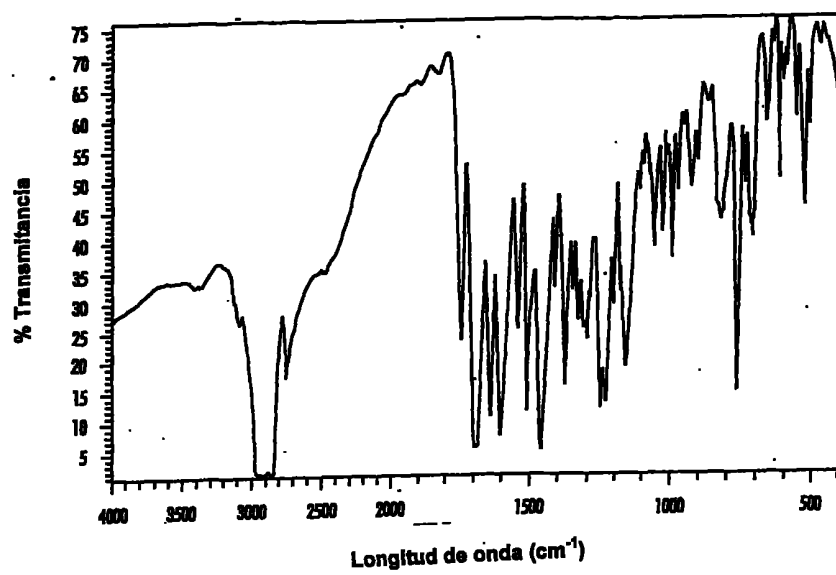
Fig.1 Espectro Infrarojo del Clorhidrato.
