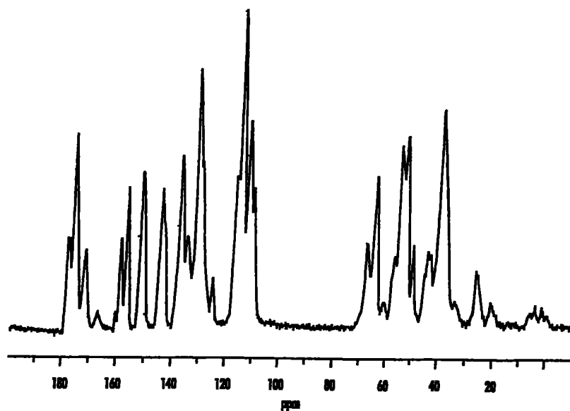
Fig 4 Espectro RMN ^{13}\text{C} en Estado Sólido del Clorhidrato
