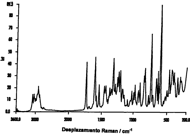
Fig 2 Espectro Raman del Clorhidrato
