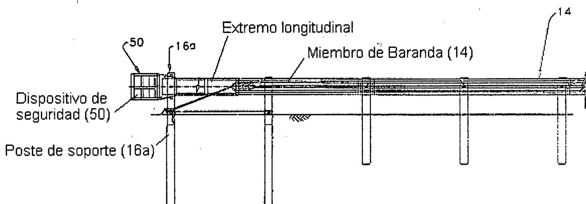
Figura 1 del documento D1 US 6109597
