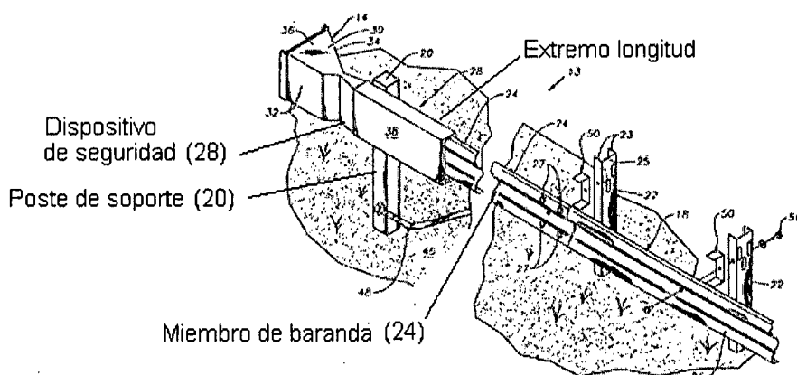
Figura 5 de la solicitud en estudio
