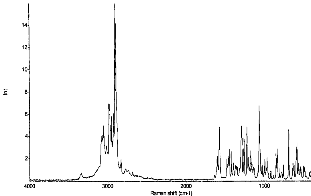
Espectro Raman (1)
