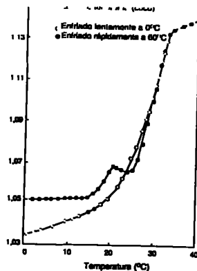
Fig. 83-7. Curvas dilatométricas de acetato de soborano (casco) con enfriamiento lento y rápido.
