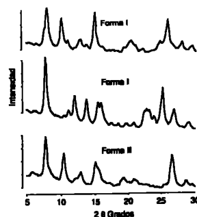
Fig. 83-9. Difractogramas de rayos X para las Formas I, II y III de SKAP 30097.
