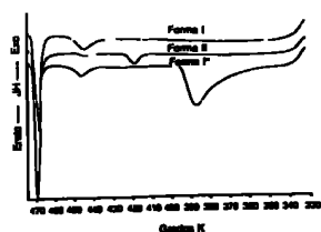
Fig. 83-8. Termogramas para las Formas I, II y III de SKAP 30097.
