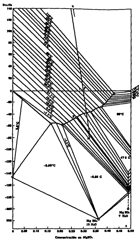
Fig. 30.48. Diagrama entalpía/concentración \text{MgSO}_4 - \text{H}_2\text{O} (B1)
