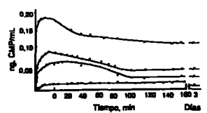
Fig. 83-13. Curvas de disolución del polimorfo C del palmitato de clorfeniramina en alcohol absoluto al 50% y en agua a 30°C, 20°C, 15°C y 0°C. Soluto: 30°C, O—O; 20°C, Δ—Δ; 15°C, □—□; 0°C, —.
