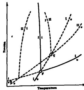
Fig. 30.44 Sistema monotrópico.
