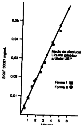
Fig. 83-11. Comportamiento de disolución de las Formas I y II de SKAF 30087 en el líquido plástico artificial.
