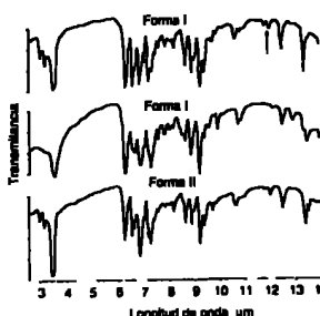
Fig. 83-10. Espectros infrarrojos de las Formas I, II y III de SKAP 30097.
