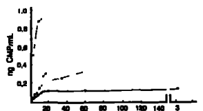
Fig. 83-14. Curvas de disolución de los polimorfos A y B del palmitato de clorfeniramina en alcohol absoluto al 50% y en agua a 30°C y 15°C. Soluto: polimorfo A, 30°C, O—O; polimorfo B, 30°C, Δ—Δ; polimorfo A, 15°C, □—□; polimorfo B, 15°C, —.
