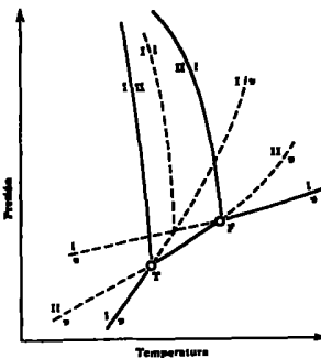
Fig. 30.43 Sistema enantiotrópico
