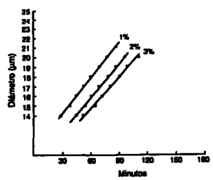
Fig. 83-4. Velocidad de crecimiento de la Forma I de una droga experimental en suspensión acuosa.
