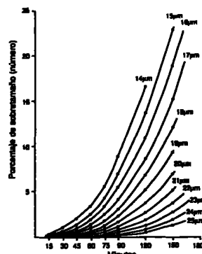
Fig. 83-4. Cambio en el porcentaje remanente en función del tiempo para una suspensión acuosa de la Forma I de una droga experimental.
