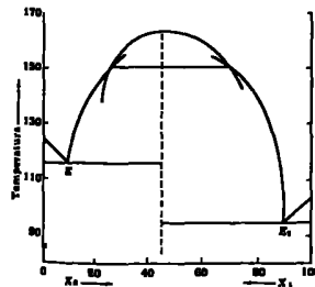
Fig. 30.42 Diagrama de composiciones para 1-3-5 trinitrobenzénico (A) y fenastreno (B) mostrando el polimorfismo del compuesto de adición (117).
