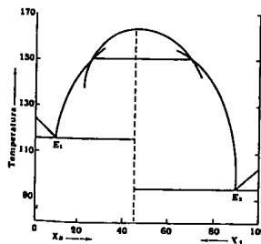
Fig. 30.45. Diagrama de composición para 1:3.5. Entre buteno (A) y fenantreno (B) mostrando el polimorfismo del compuesto de adición (117).
