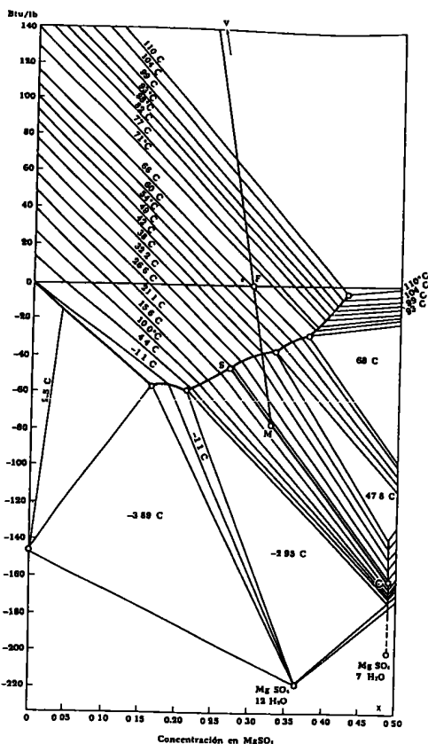
Fig 30 42 Diagrama entalpia/concentración MgSO_4 - H_2O (81)
