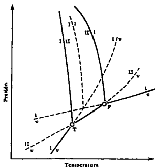
Fig. 30.43. Sistemas enantiotrópicos.
