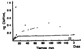
Fig. 83-14 Curvas de disolución de los polimorfos A y B del palmitato de cloramfenicol en alcohol i-butílico al 15% y en agua a 10°C y 15°C. Símbolos: polimorfo A: 10°C: ○—○; 15°C: ●—●; polimorfo B: 10°C: ▲—▲; 15°C: ▼—▼.
