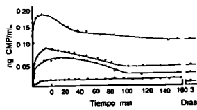
Fig. 83-13 Curvas de disolución del polimorfo C del palmitato de cloramfenicol en alcohol i-butílico al 15% y en agua a 10°C, 15°C y 20°C. Símbolos: 10°C: ○—○; 15°C: ●—●; 20°C: ▲—▲.
