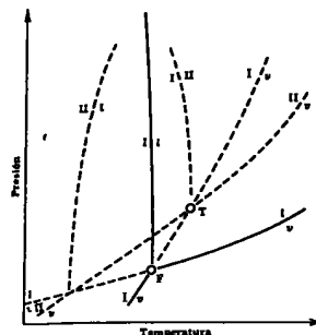
Fig. 30.44. Sistemas monotrópicos.
