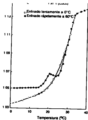
Fig. 83-7. Curvas dilatométricas, acetato de teobroma (cacao) con enfriamiento lento y rápido.
