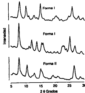
Fig. 83-9. Difractogramas de rayos X para las Formas I y II de SK&F V097.
