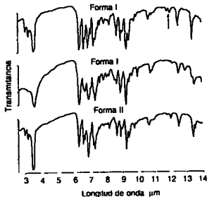
Fig. 83-10. Espectros infrarrojos de la Forma I y II de SK&F V097.
