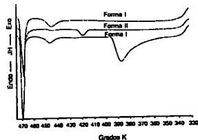
Fig. 83-8. Termogramas para las Formas I y II de SK&F V097.
