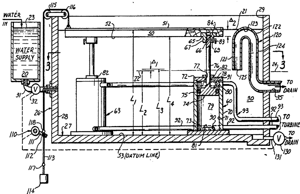
Fig. 1 del documento US 3961480
