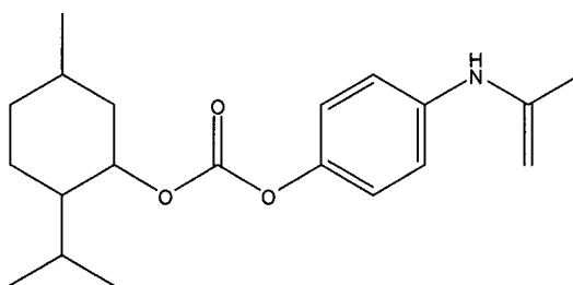
2-isopropil-5-metilciclohexil 4-(prop-1-en-2-ilamino)fenil carbonato
