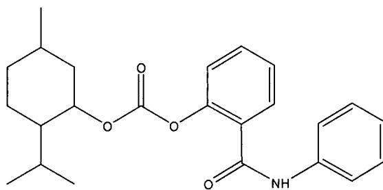
2-isopropil-5-metilciclohexil 2-(fenilcarbamoyl)fenil carbonato
