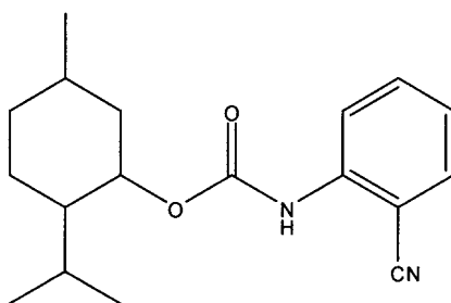
2-isopropil-5-metilciclohexil 2-cianofenil carbamato
