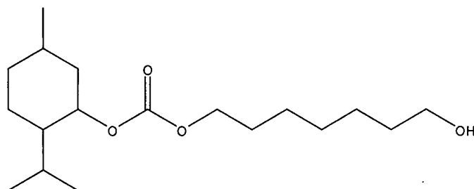
7-hidroxiheptil 2-isopropil-5-metilciclohexil carbonato
