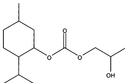
2-hidroxipropil 2-isopropil-5-metilciclohexil carbonato
