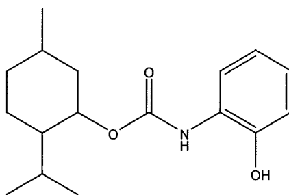
2-isopropil-5-metilciclohexil 2-hidroxifenil carbamato,
