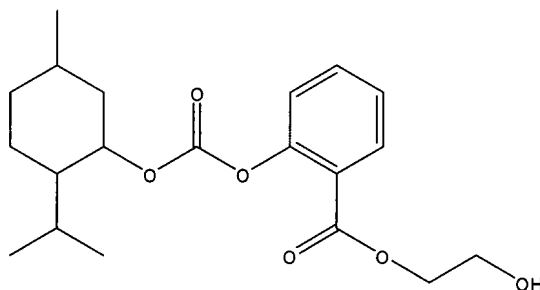
2-hidroxietil 2-((2-isopropil-5-metilciclohexiloxi)carboniloxi benzoato
