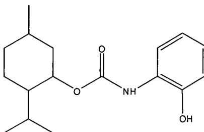
2-isopropil-5-metilciclohexil 2-hidroxifenil carbamato
