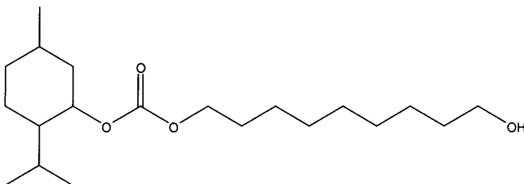
7-hidroxiheptil 2-isopropil-5-metilciclohexil carbonato
