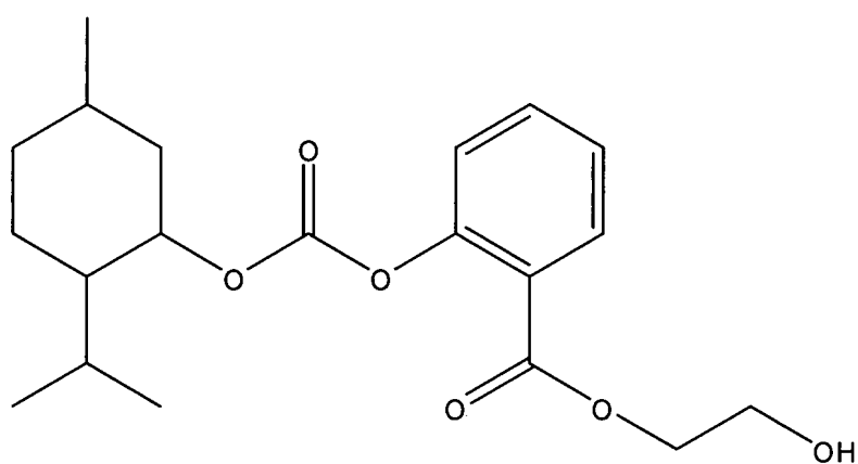
2-hidroxietil 2-((2-isopropil-5-metilciclohexiloxi)carboniloxi benzoato
