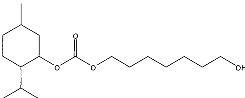
7-hidroxihetil 2-isopropil-5-metilciclohexil carbonato
