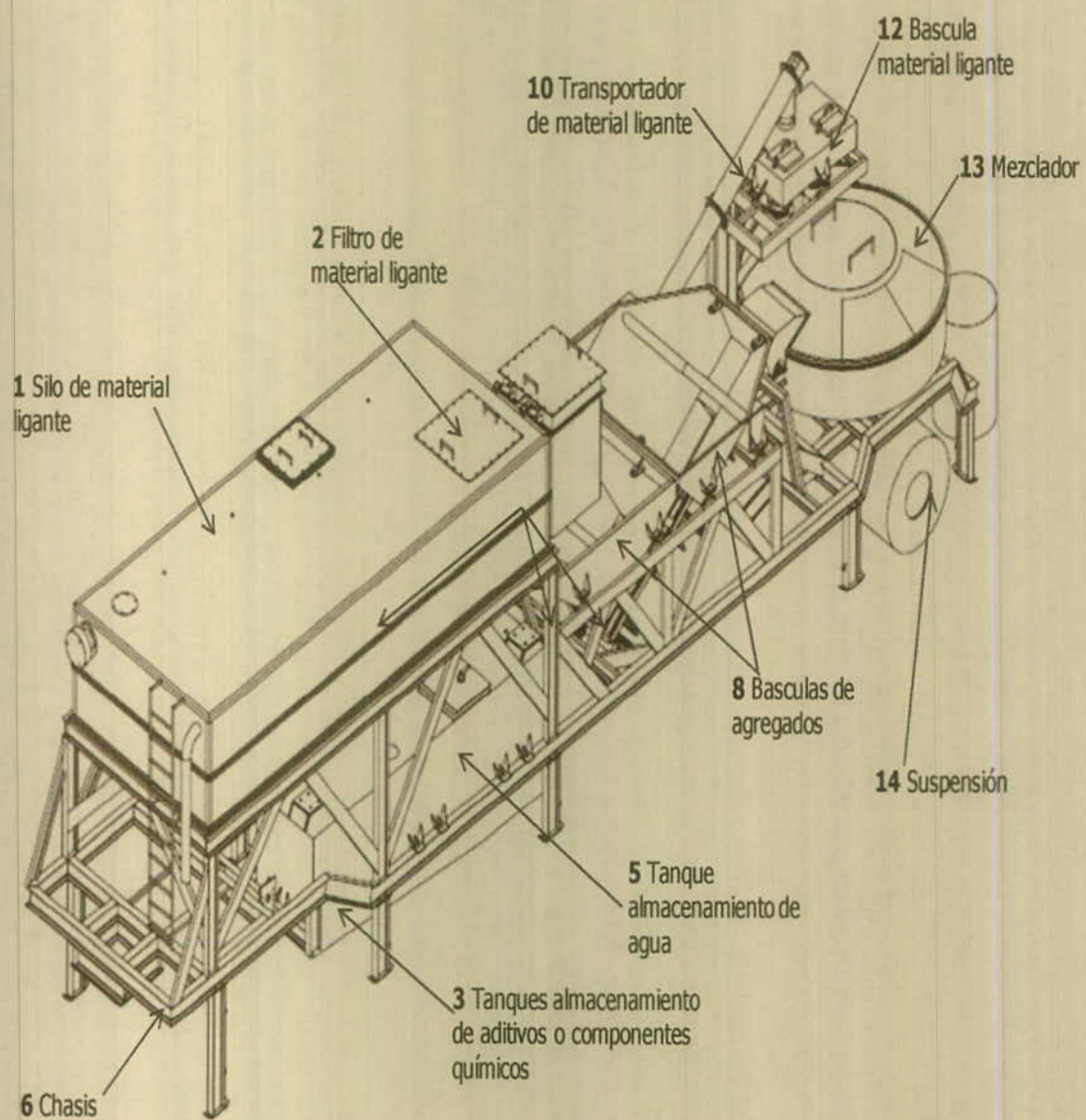
Figura 7. Vista isométrica del equipo.
