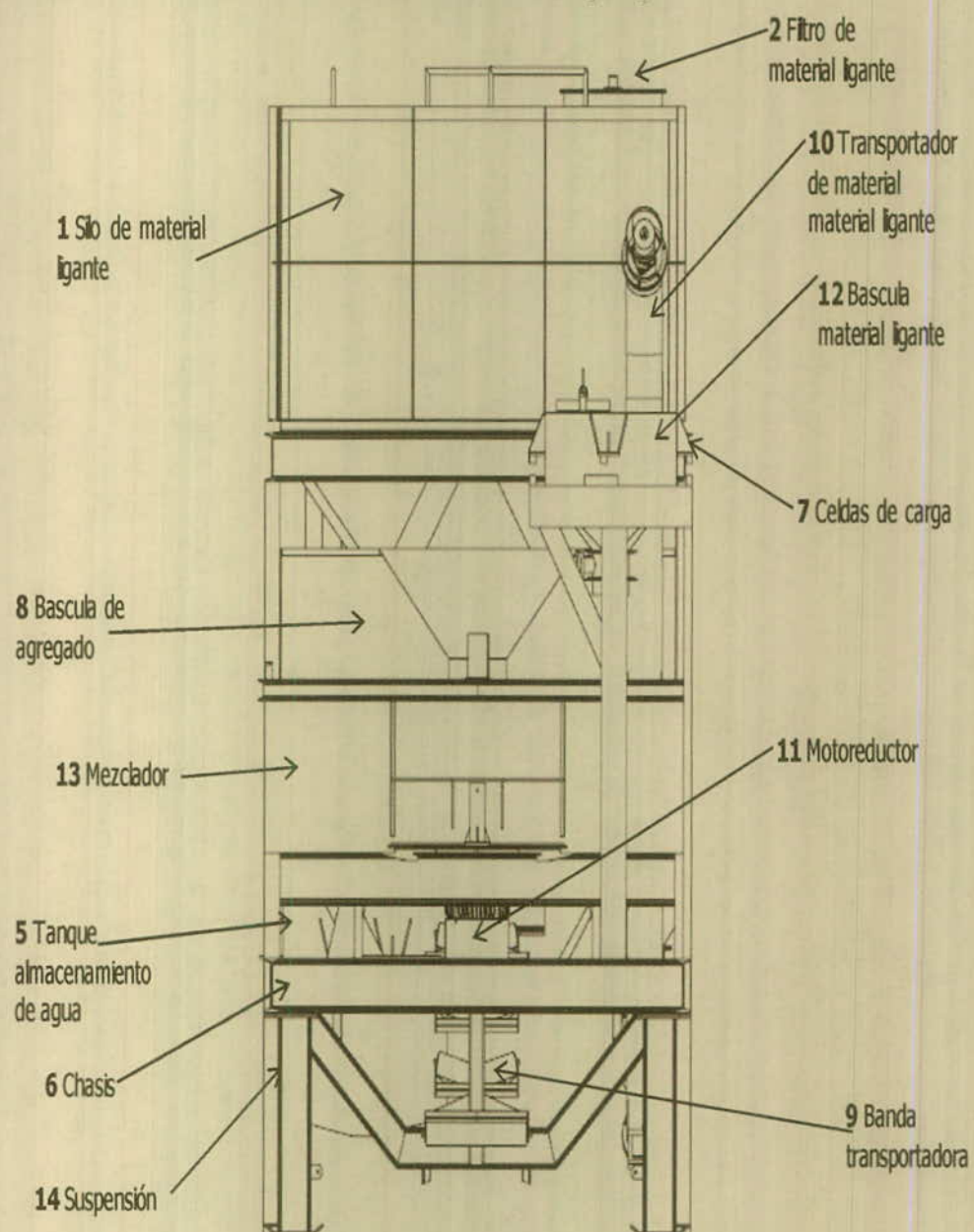
Figura 5. Vista Trasera del equipo
