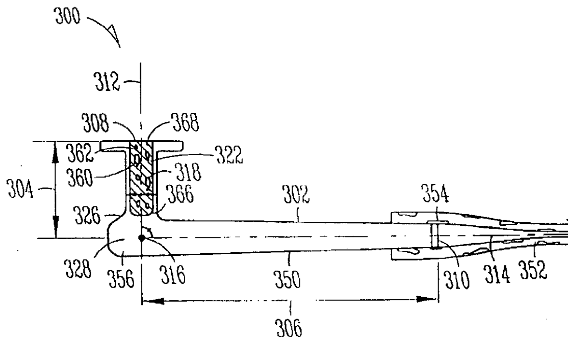
SECTION 3B-3B
