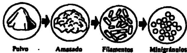
FIGURA 2.32. Diagrama secuencial de un proceso de extrusión/esferonización.
