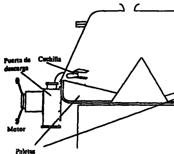
FIGURA 2.30. Esquema de un mezclador/granulador de tipo Z.
