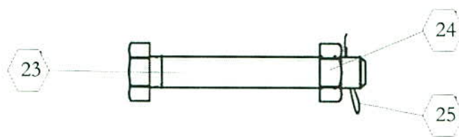
Figura No. 23. Diseño del eje de la placa de anclaje del tensor.
