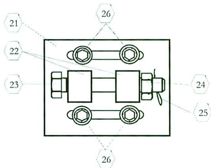
Figura No. 20. Vista superior de la placa de anclaje.
