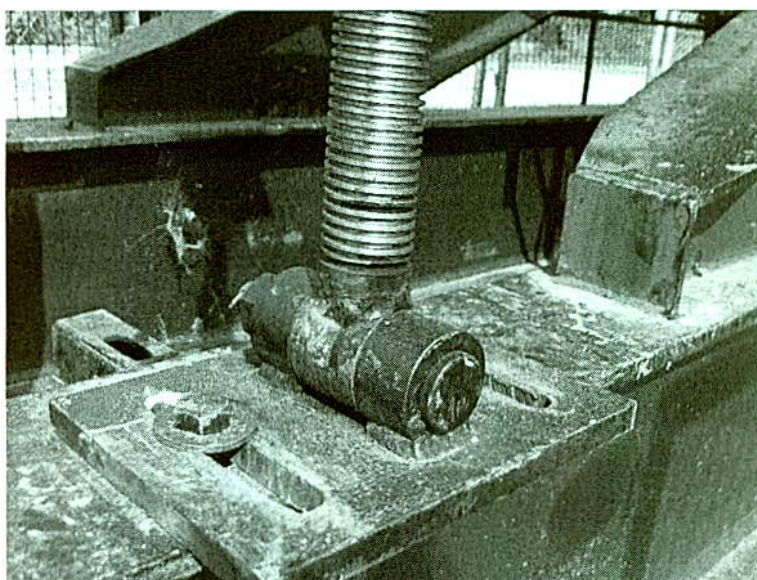
Figura 30, placa de anclaje del tensor
