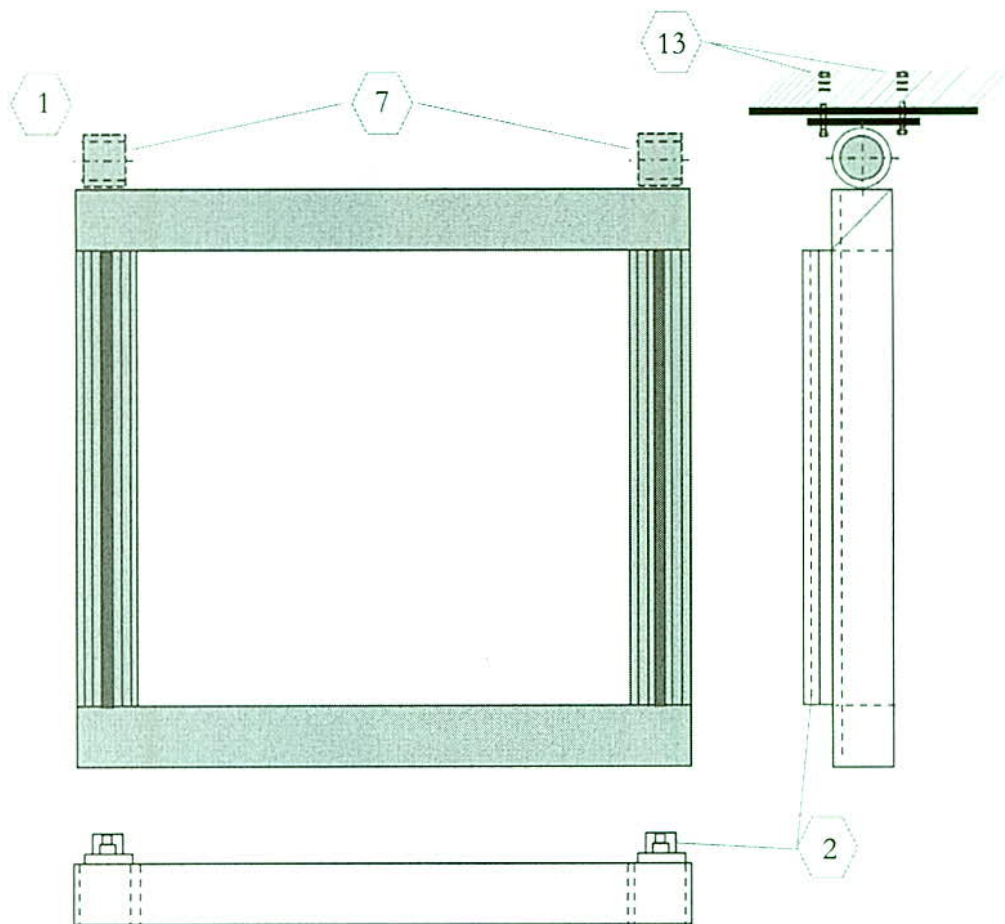
Figura 26, Plano de la mesa del motor rediseñada.
