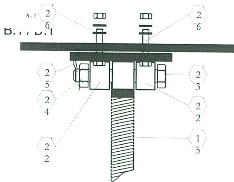
Figura No. 19. Diseño de las placas de anclaje.
