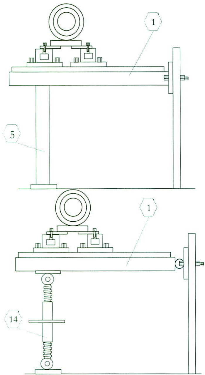
Figura No. 24. Propuesta para la mesa del motor ubicada dentro de la estructura.
