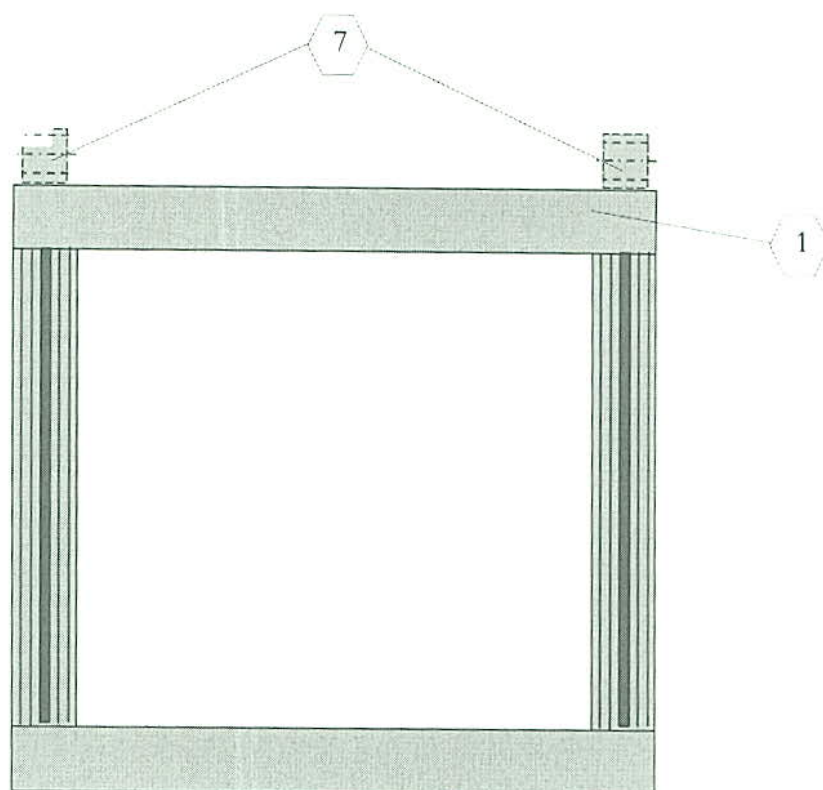
Figura No. 11. Vista superior de la mesa del motor con los bujes de anclaje montados.
