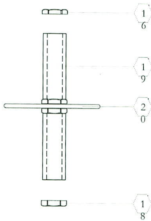
Figura No. 17. Cuerpo del tensor y tuercas de los tornillos.
