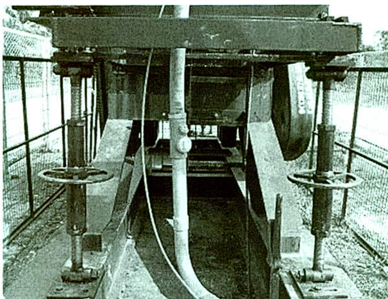
Figura 28, Vista frontal de la mesa del motor del motor rediseñada en una unidad de bombeo mecánico.
