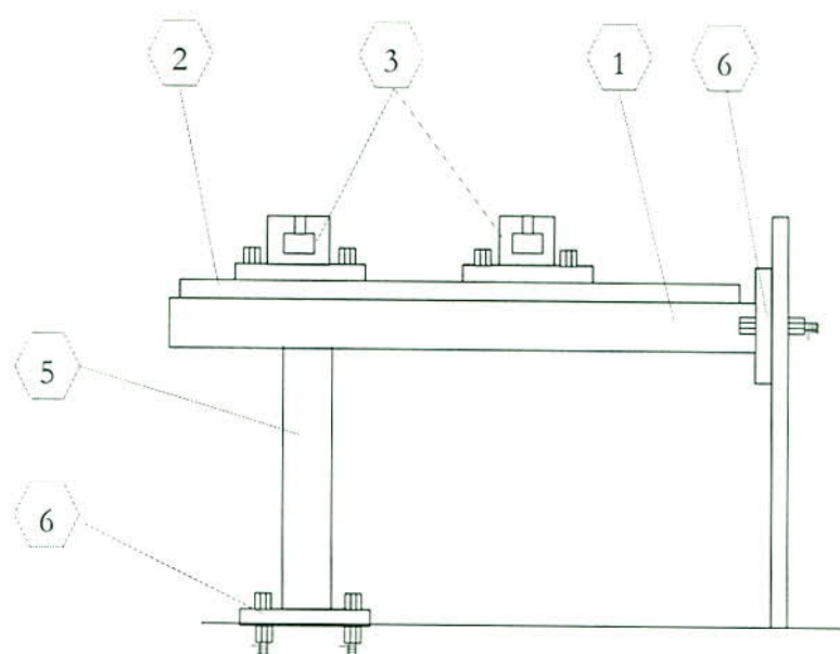
Figura No. 3, Vista lateral de la mesa del motor eléctrico esquematizando los dos dispositivos originales de apoyo o anclaje.
