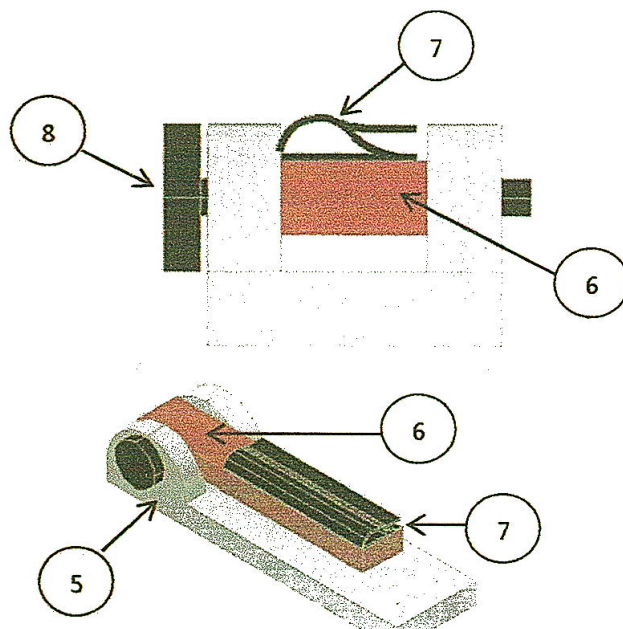
Figura 2, Detalle (4)
