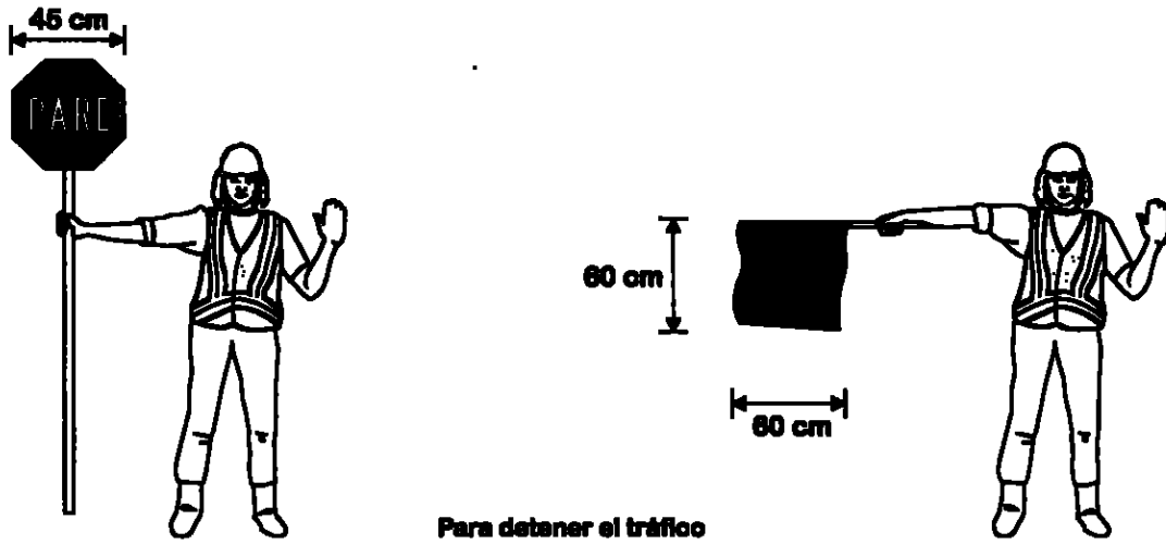
Figura 4.9 Bandereros y uso de banderas y paletas
