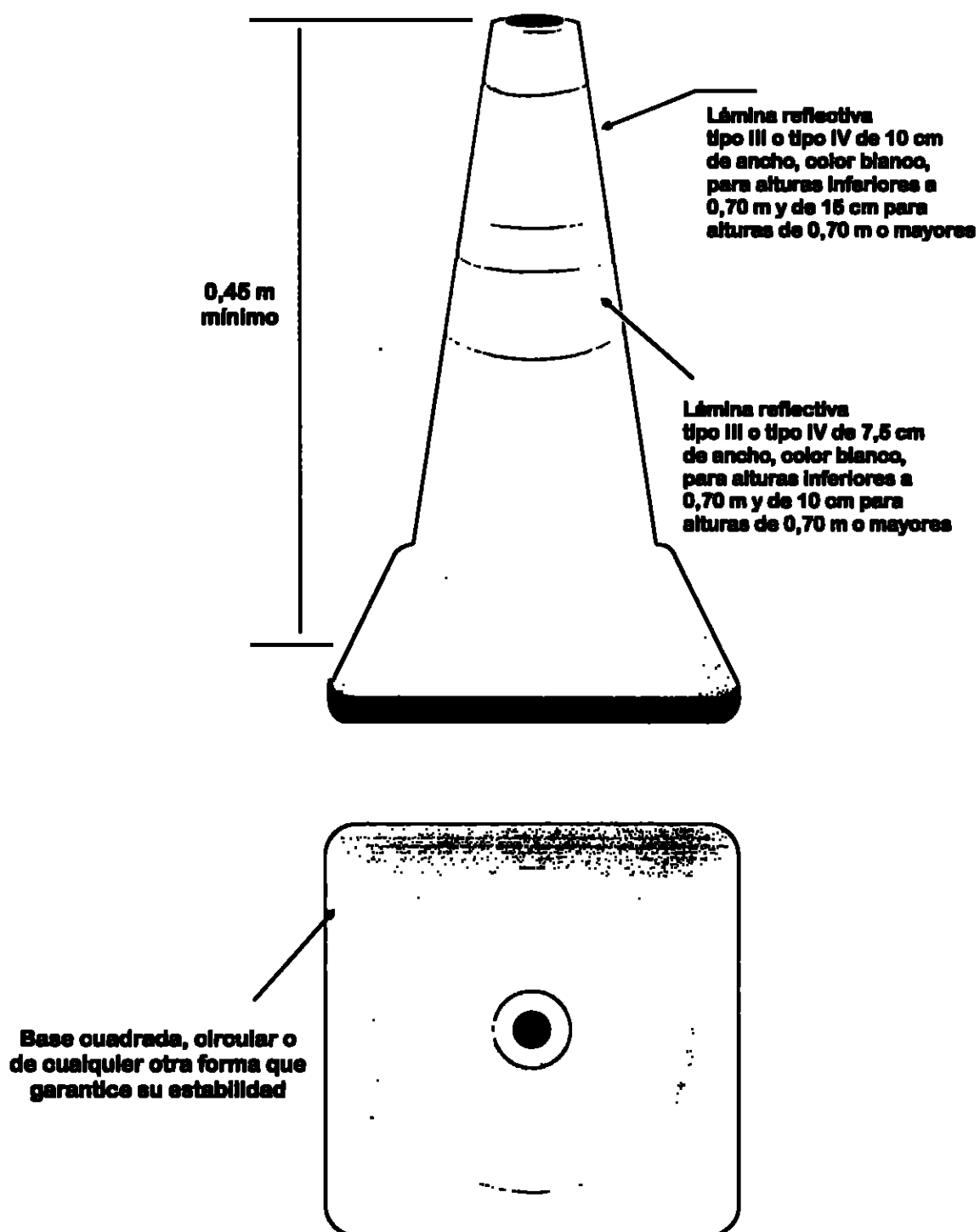
Figura 4.2 Conos
