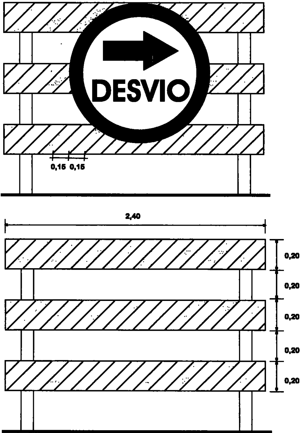
Figura 4.1 Barricadas (dlmensiones en metros)
