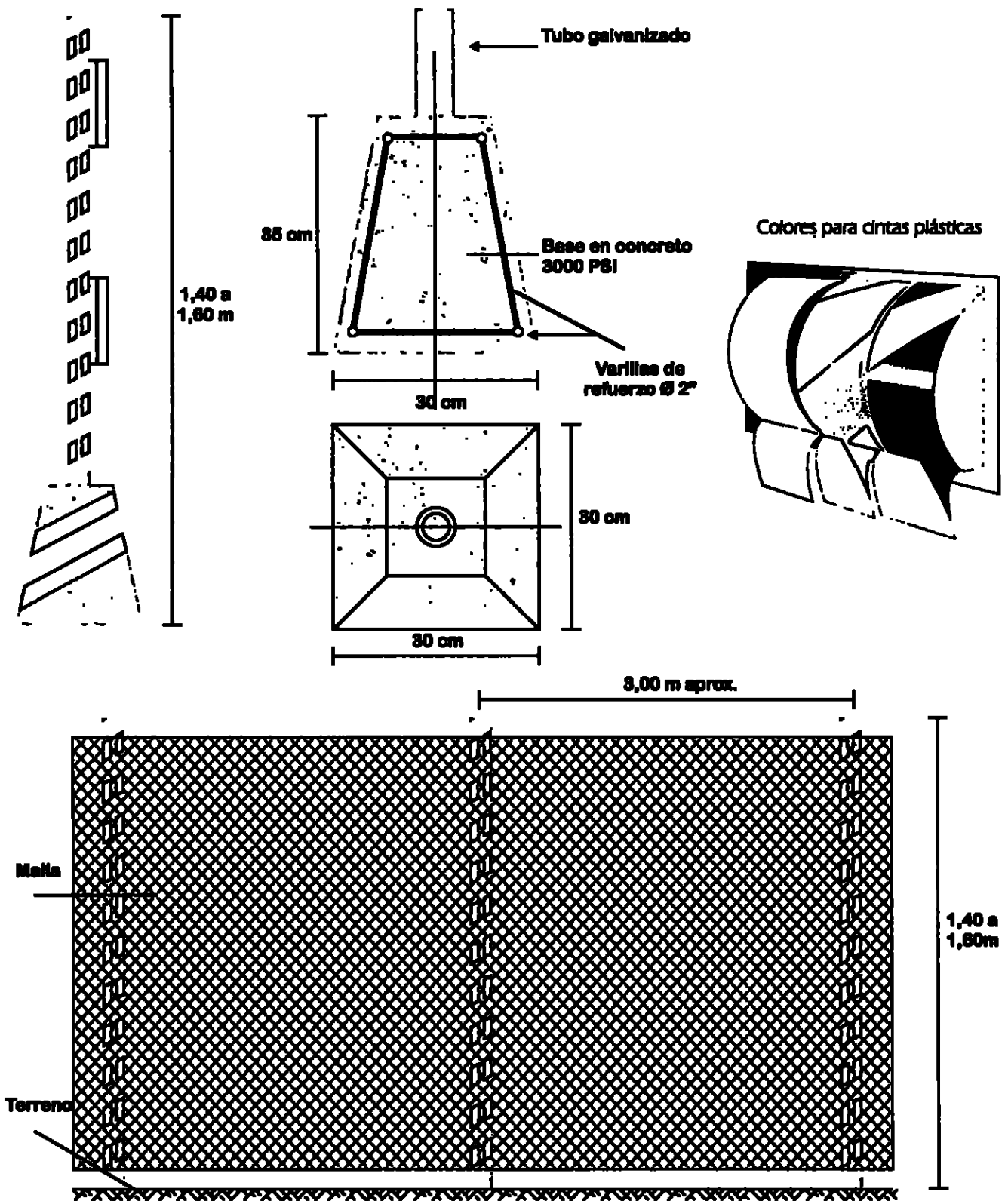
Figura 4.6 Tabiques, cintas plásticas y mallas
