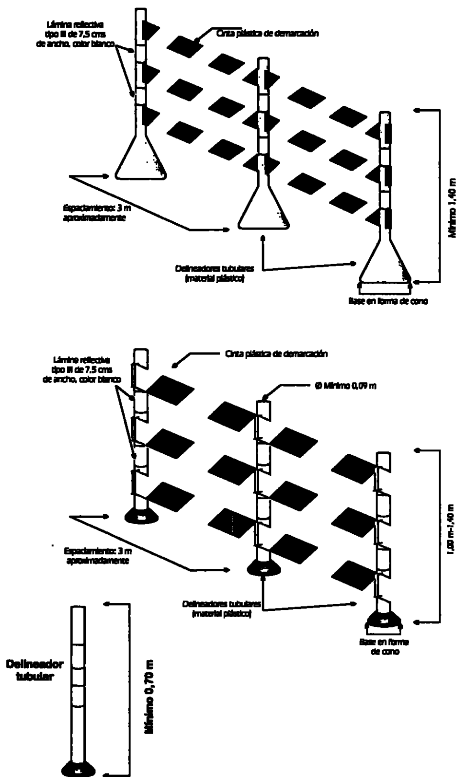
Figura 4.3 Delineadores tubulares
