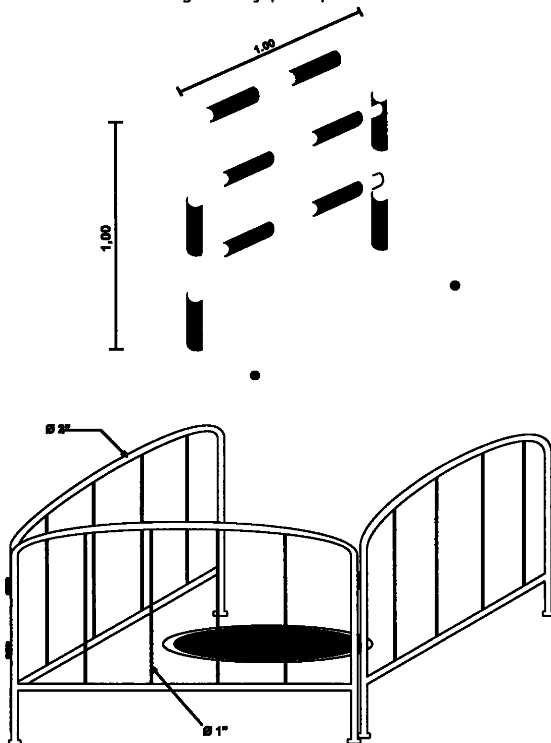
Figura 4.7 Reja portátil peatonal
