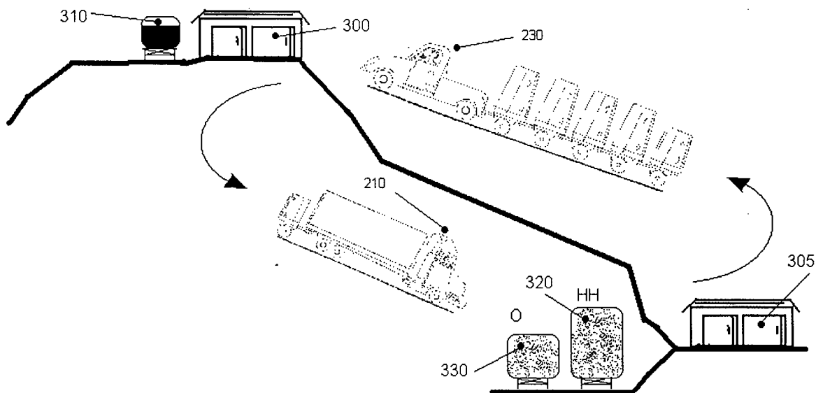
Figura 2. Sistema de producción de hidrógeno y oxígeno.
