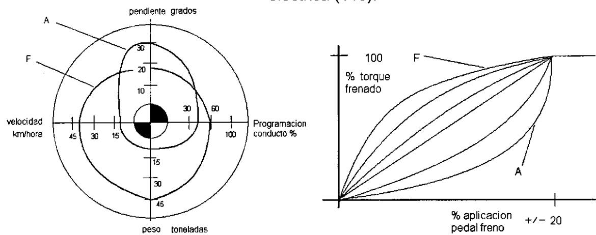
Figura 6. Izquierdo, explicación grafica de cómo el PIC (140) determina la curva de acción del frenado del generador (120). Derecha, diferentes curvas de acción de frenado.
