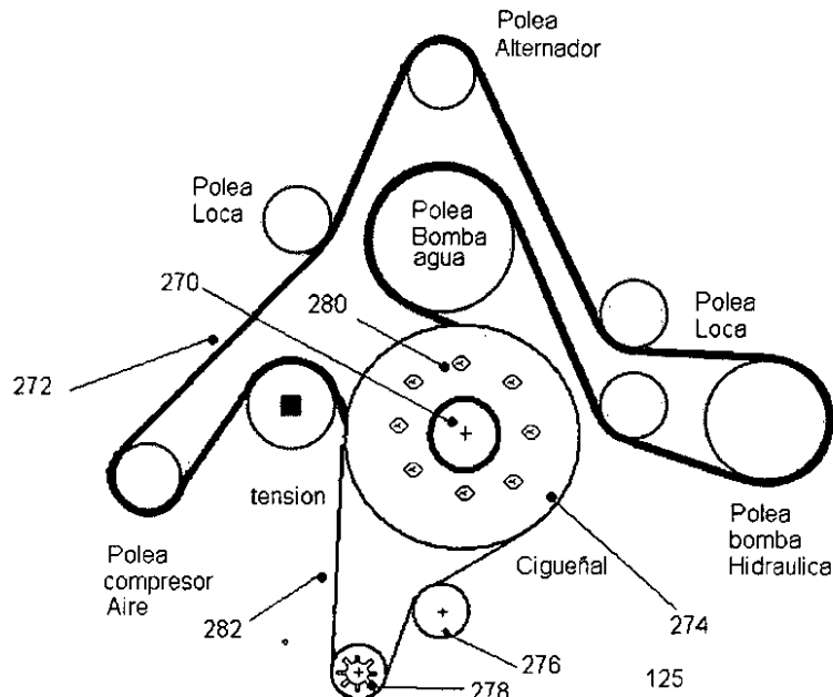
Figura 5. Sistema de transmisión movimiento de modulo de generación energía eléctrica (115).
