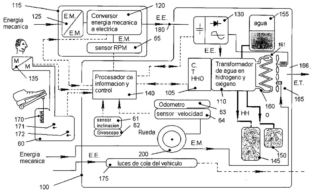
Figura 7. Esquema del equipo móvil de recuperación y producción EMRP (103).
