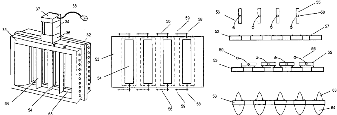
Figura 3a. Esquema de servo-válvula (32)
