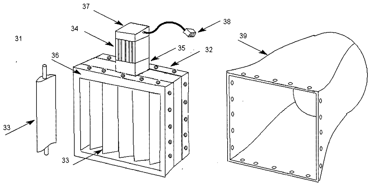
Figura 3. Esquema de servo-válvula (31)
