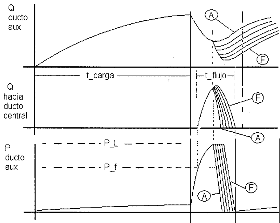
Figura 11. Variación de presión y caudal en cada convertidor (20) según demanda.
