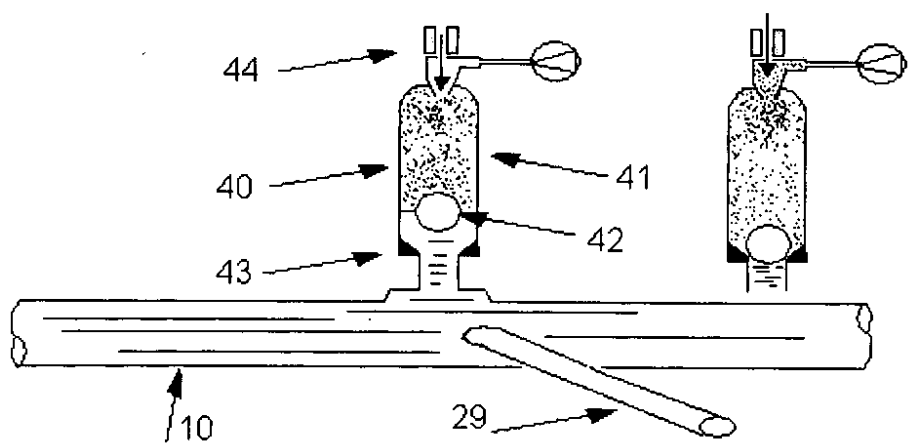
Figura 9. Atenuador de variaciones de presión (40).
