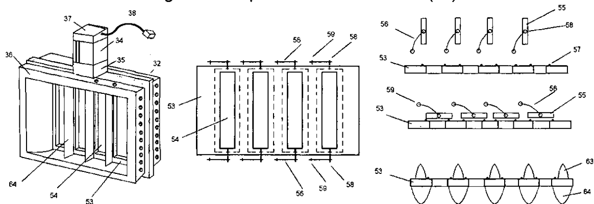
Figura 3ª. Esquema de servo-válvula (32)
