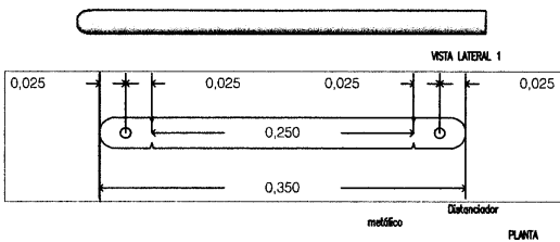
PLANTA
