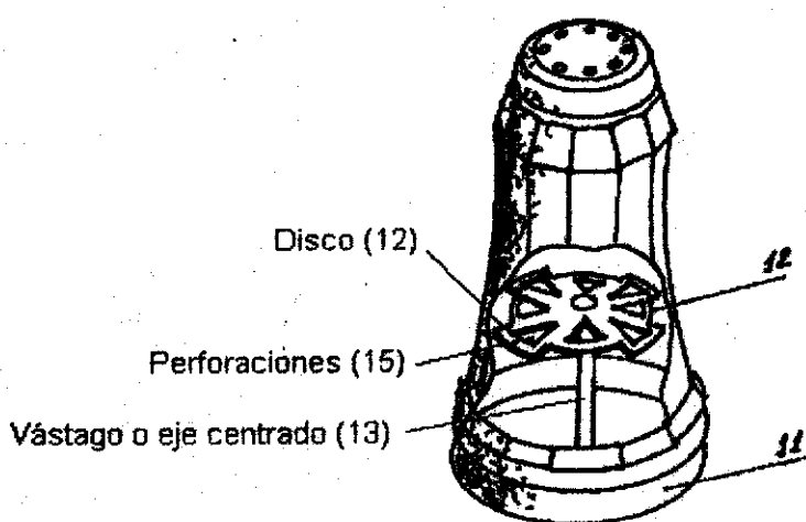
Figura 1 de la solicitud en estudio
