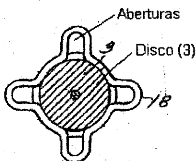
Figura 9 del documento D1 US 1931087
