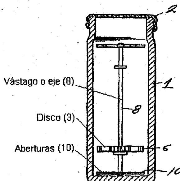
Figura 3 del documento D1 US 1931087
