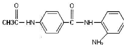
Estructura química de CI-94 (acetyldinaline)
