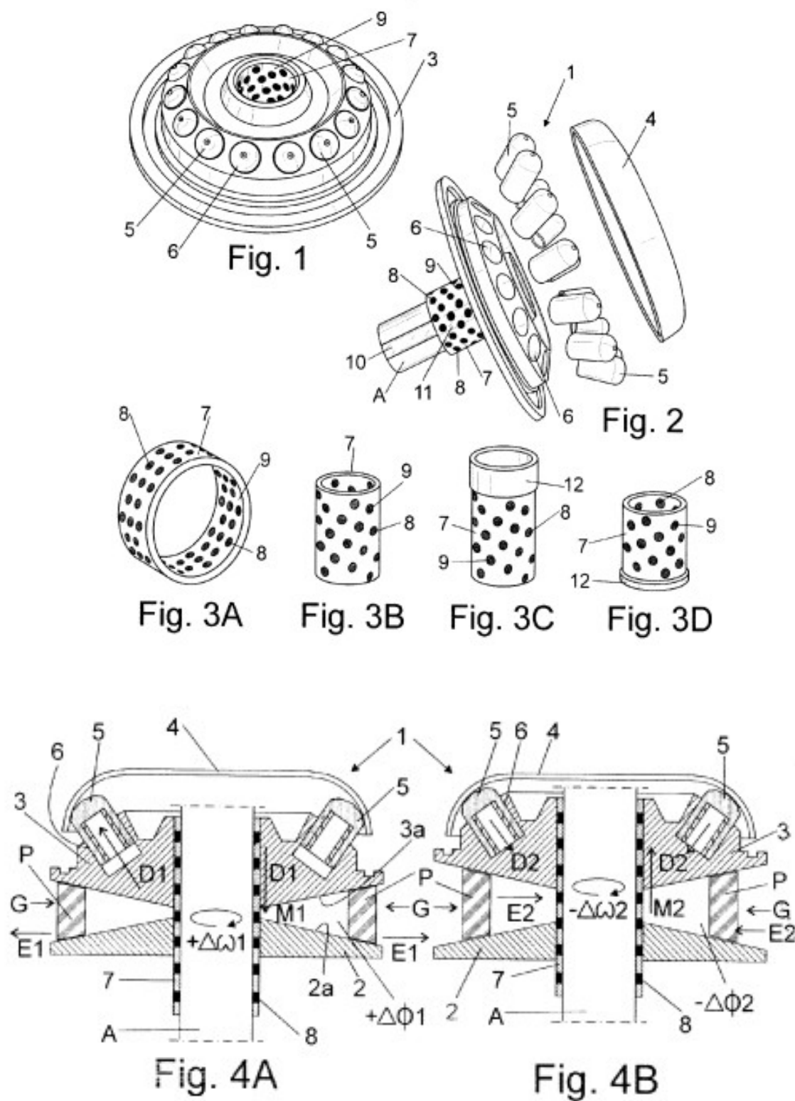
Figura 1, 2, 3a, 3b, 3c, 3d, 4a y 4b del documento D1 ES 1069285
