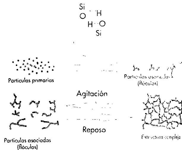
FIGURA 4.32. Representación esquemática de la interacción que se produce entre las partículas de Aerosil®. La asociación lleva a la formación de flóculos que en reposo crean una estructura compleja. La agitación permite recuperar la suspensión original. El sistema presenta propiedades tixotrópicas.
