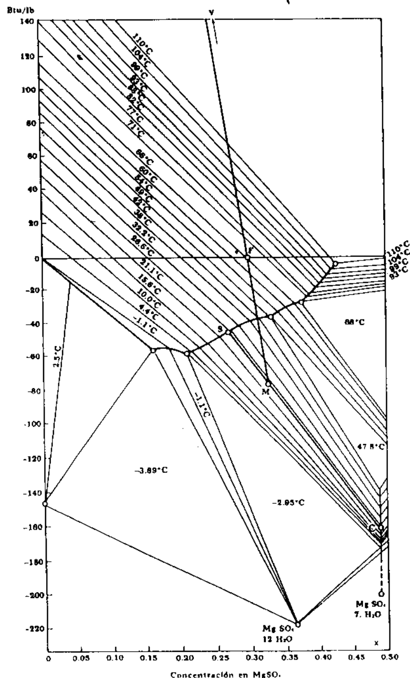
Fig. 30.42. Diagrama entalpía-concentración. MgSO_4 - H_2O (91).
