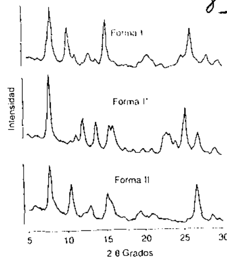
Fig. 83-9. Difractogramas de rayos X para las Formas I, I' e II de SK&F 30097.
