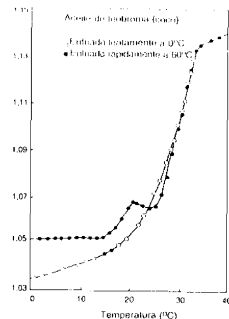
Fig. 83-7. Curvas dilatométricas, acetato de teobromina (cacao) con enfriamiento lento y rápido.
