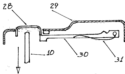
Figura 5A Corte 5-5
