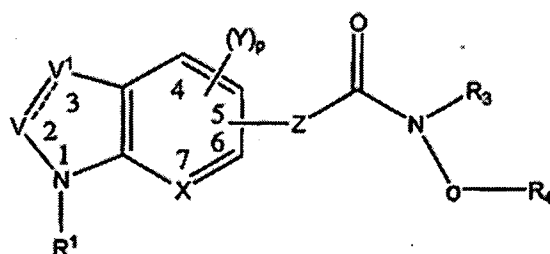
Figura 1. Estructura general de los compuestos divulgados en D5.
