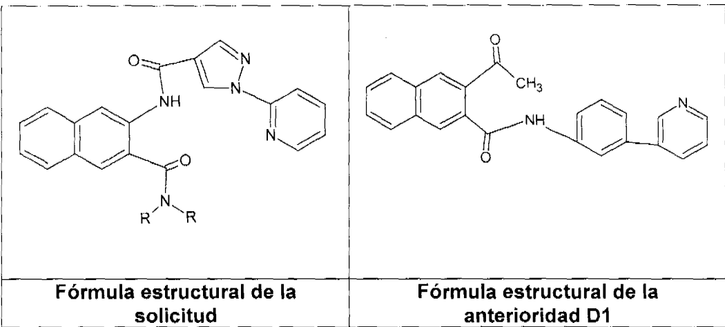
Fig.1. Comparación entre la estructura derivada de la anterioridad D1 y la estructura de la solicitud.
