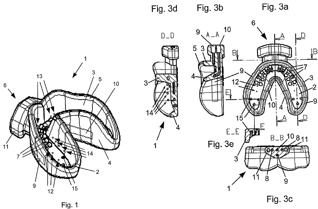
Figs. 1 y 3a-3e del documento US 2007/0184404
